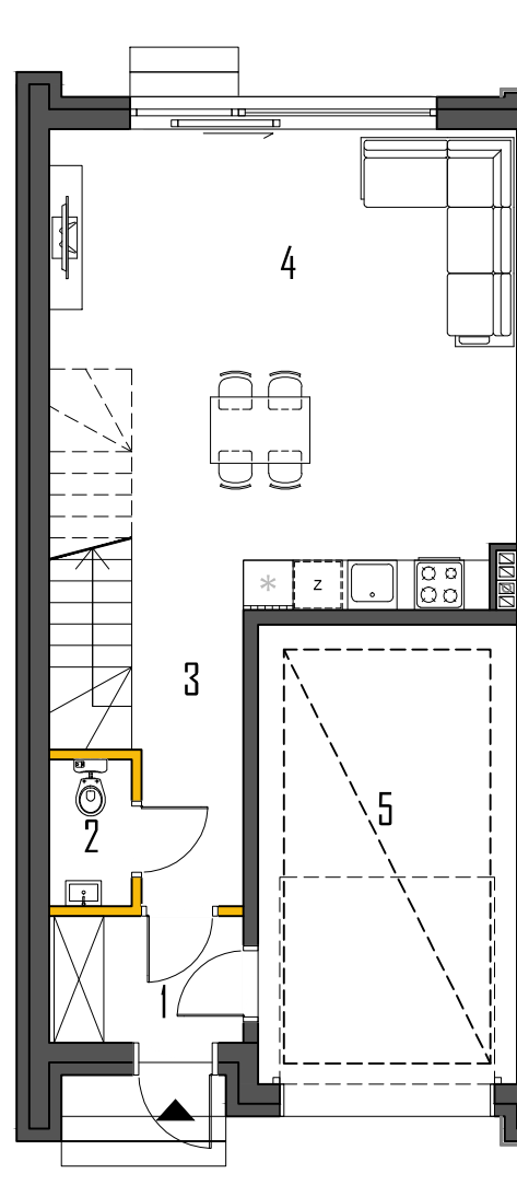
RZUT PARTERU
