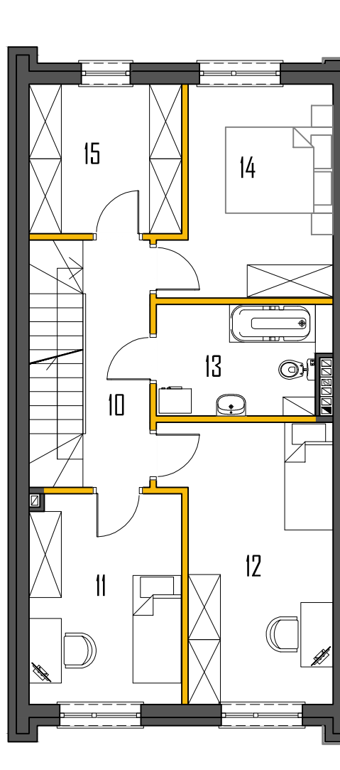
RZUT PIĘTRA
